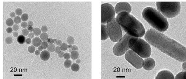
Las imágenes de microscopía de transmisión de electrones muestran partículas de óxido de hierro formados sin (redondos) y con (alargados) un surfactante presente durante su formación.
