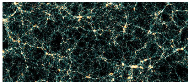
Imagen del catálogo Euclid Flagship: cada punto es una galaxia. Azul: galaxias centrales en cúmulos de materia oscura; rojo: satélites. Conjunto: distribución de masa a gran escala del Universo (cúmulos, filamentos y vacíos).
