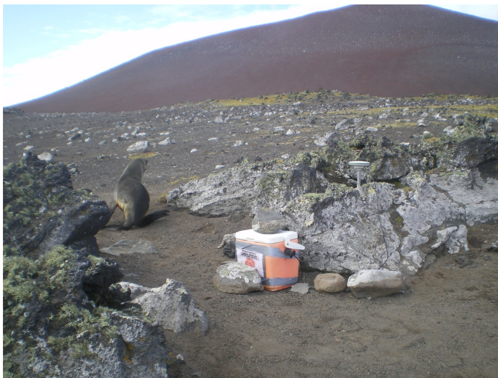
Vértice geodésico PING perteneciente a la red GNSS RGAE ubicado en la isla Pingüino.
