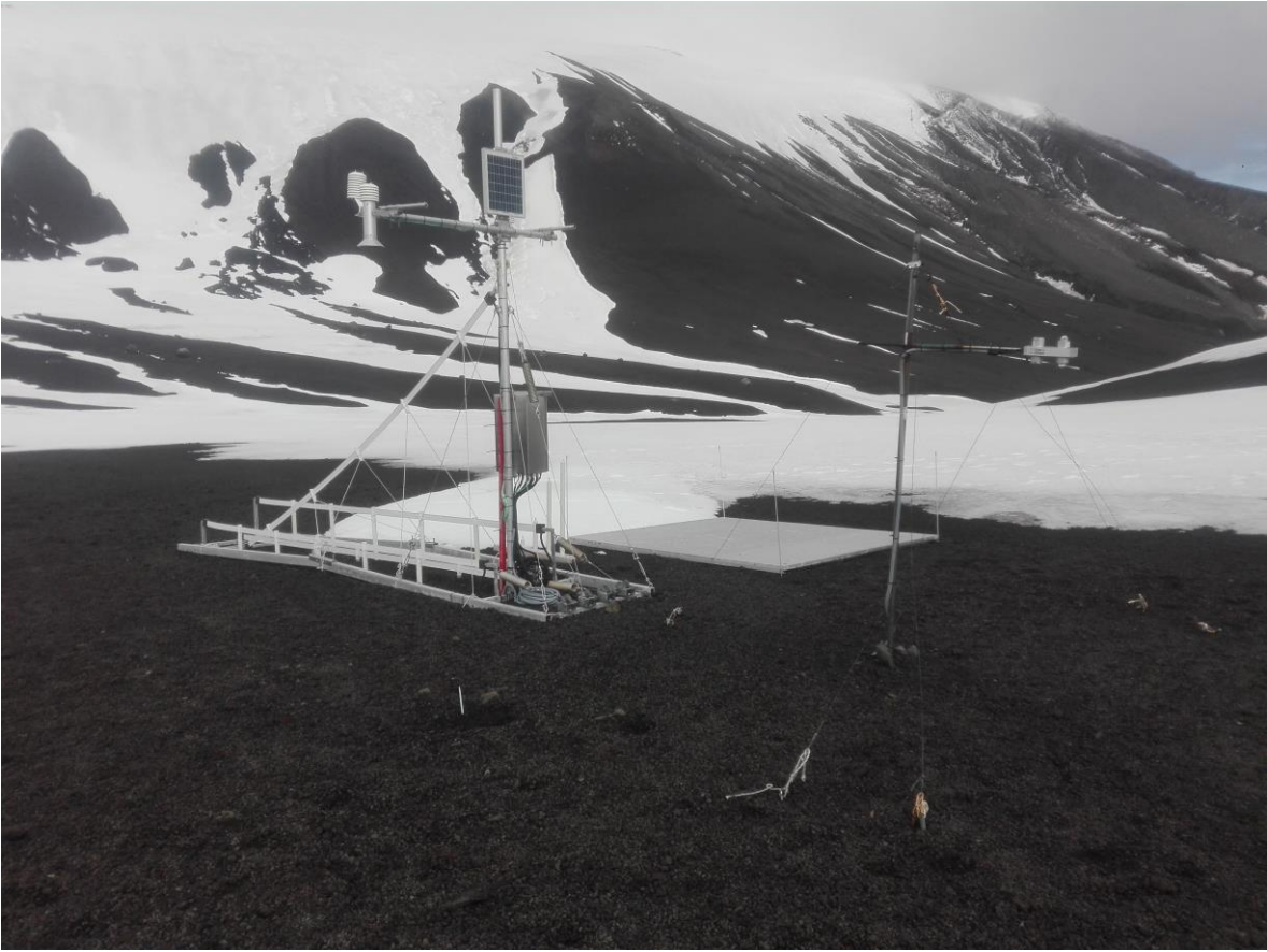
Fotografía: Algunos de los instrumentos de la red PERMATHERMAL en la isla Decepción, Antártida.
