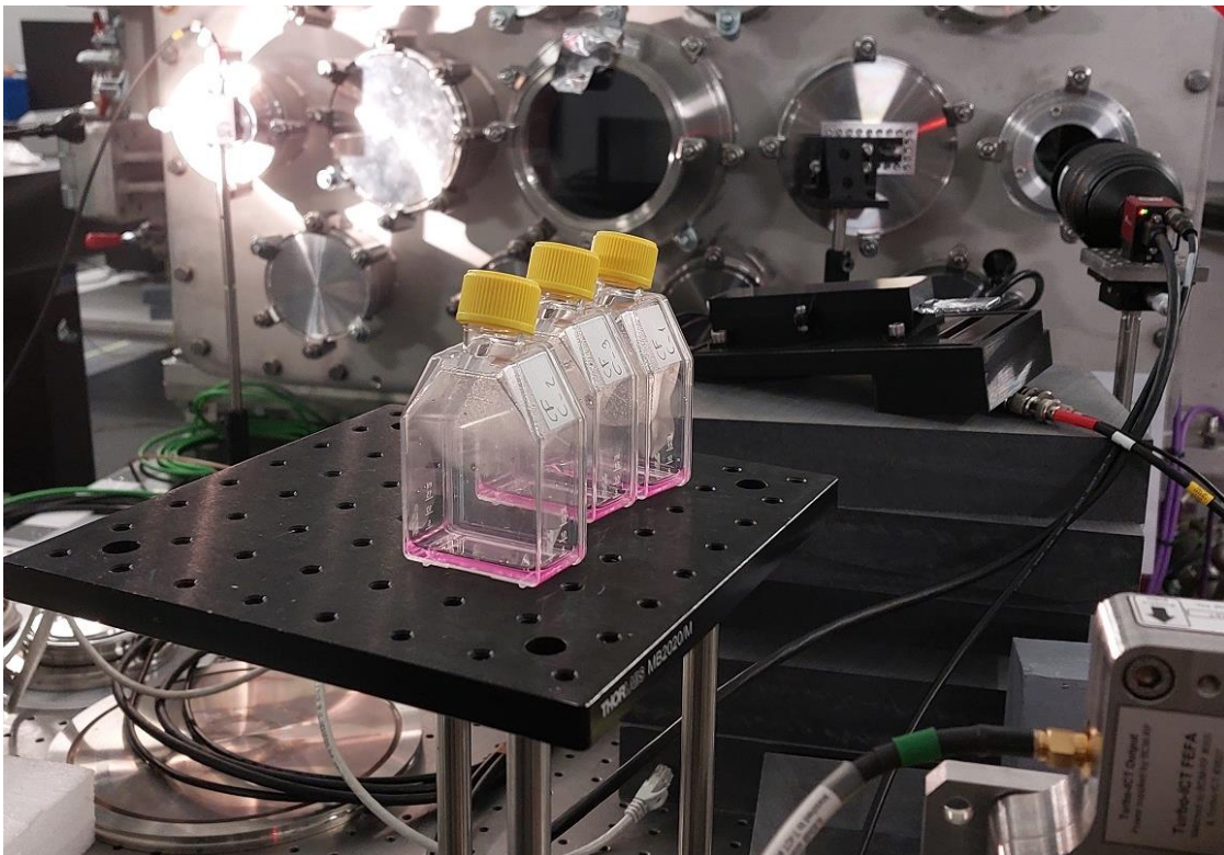
Muestras celulares y sistema de vacío del láser VEGA-3. / i3M-CLPU
